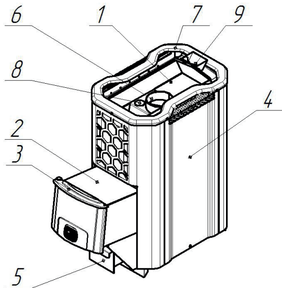
Рисунок 1 - Конструкция печи-каменки «САХАРА (2.0)»
