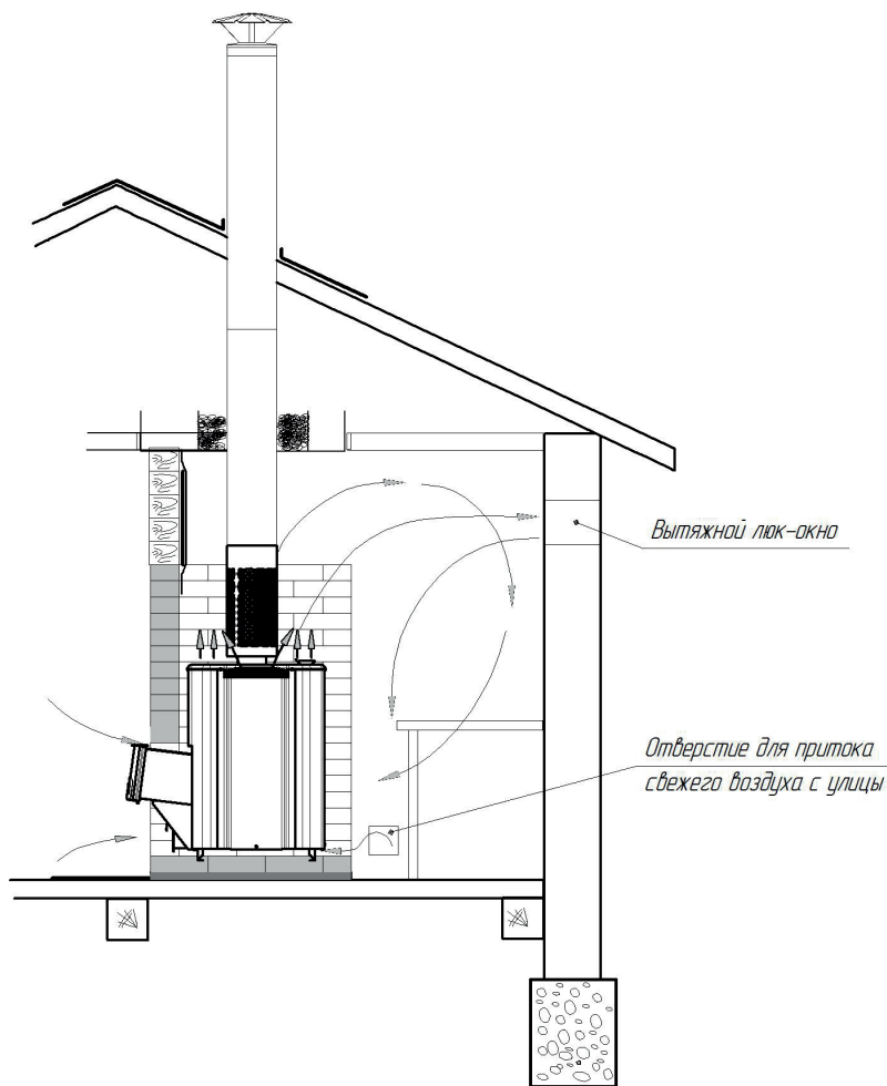
Рисунок 9 - Схема воздухообмена в парилке
