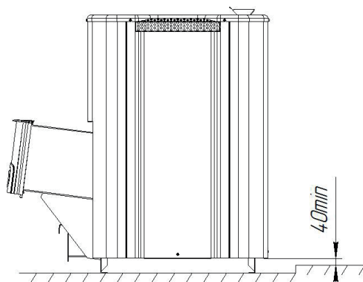
Рисунок 5 — Установка печи ниже уровня чистового пола
