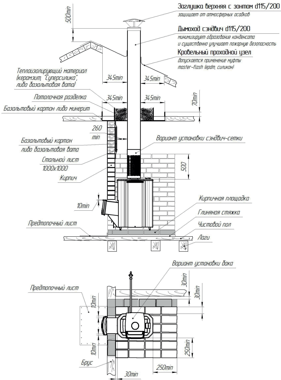
Рисунок 6 - Схема установки печи с кирпичной кладкой
