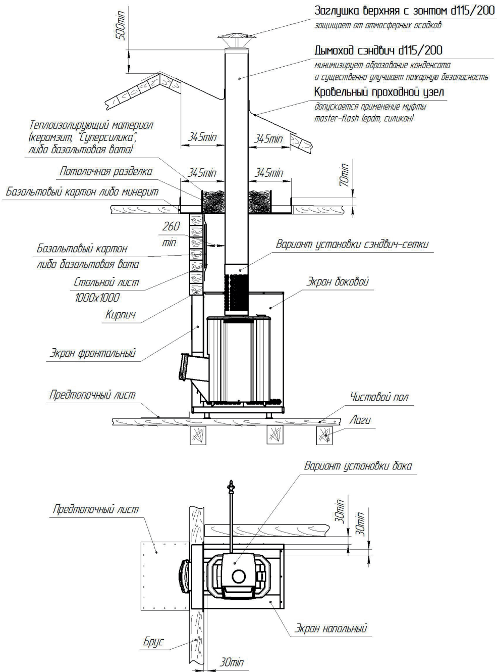
Рисунок 7 - Схема установки печи с защитными экранами
