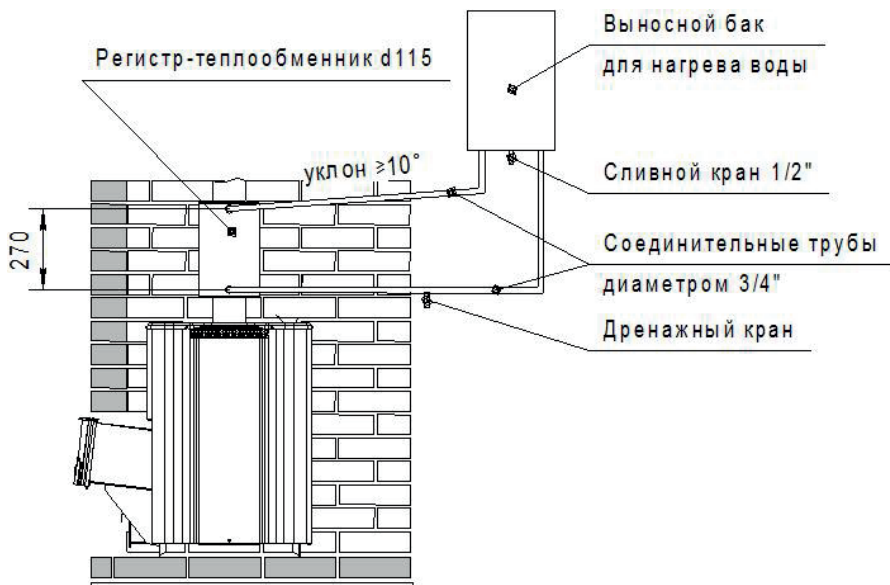
Рисунок 2 - Подключение бака с универсальным регистром-теплообменником
